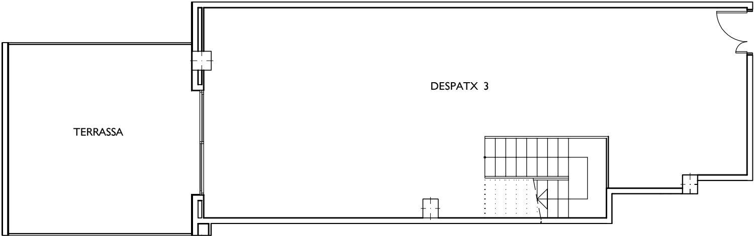
PLANTA BAIXA
